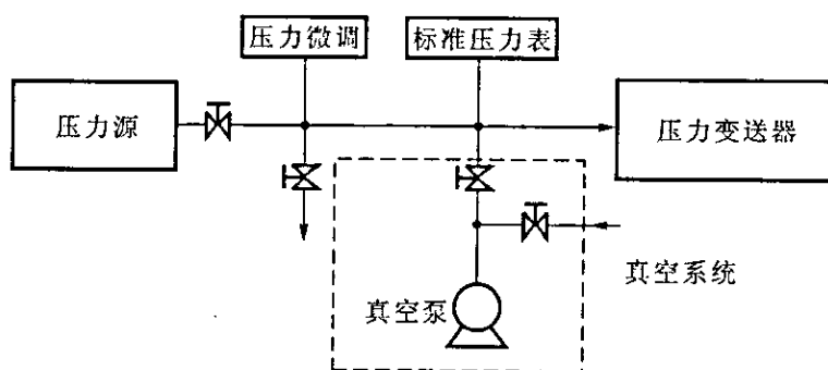
图 A-4 压力变送器输入部分的连接
