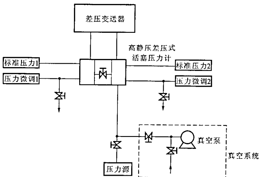
图 A-5 差压变送器输入部分的连接
